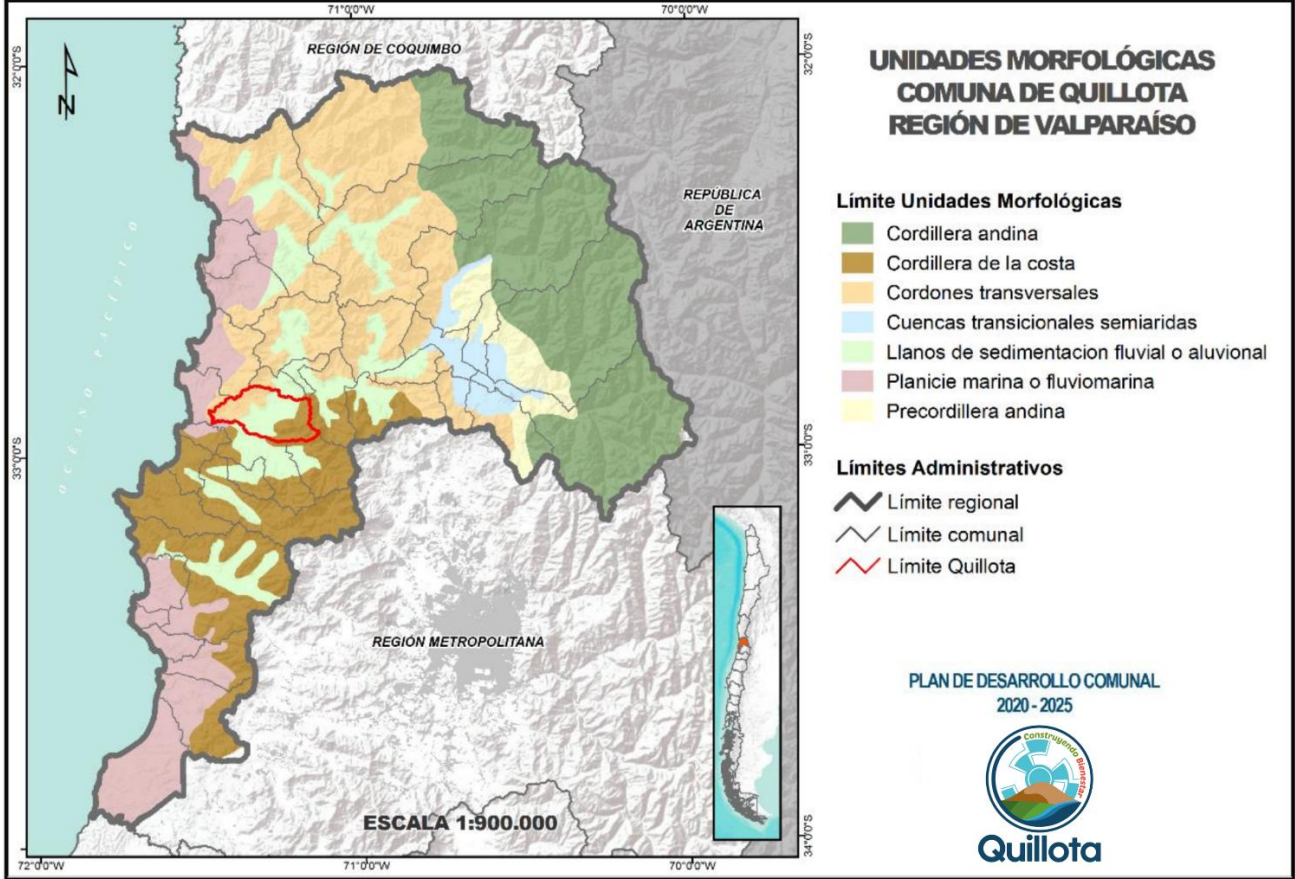
Ilustración 5: Mapa de las principales formas del relieve presentes en la Región de Valparaíso
