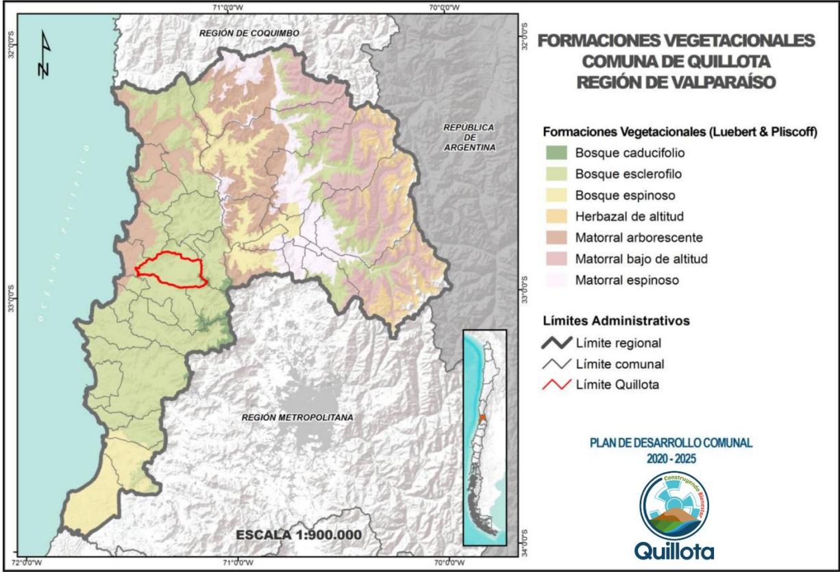
Ilustración 8: Mapa de Distribución de las distintas formaciones vegetacionales en la Región de Valparaíso
