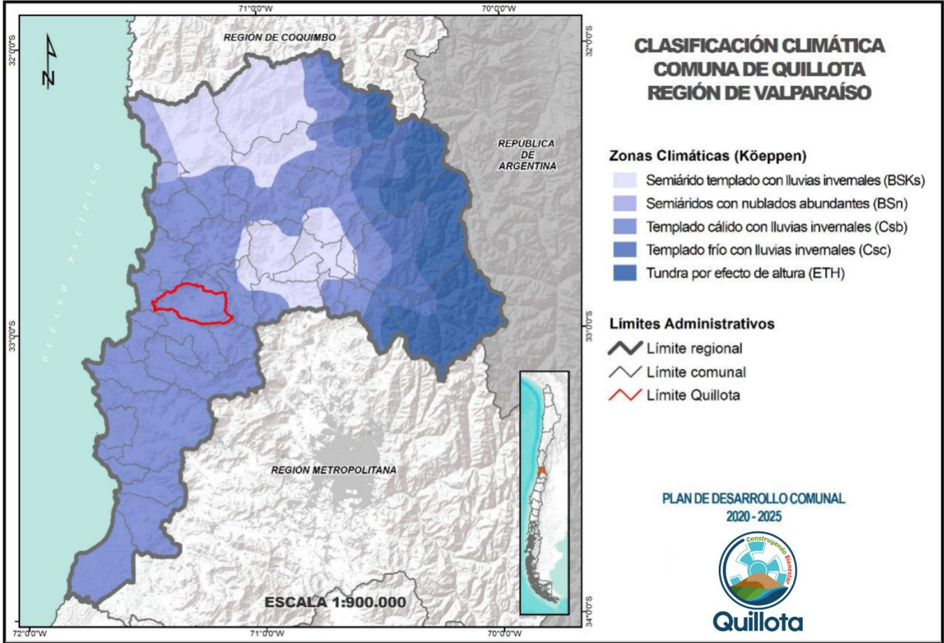
Ilustración 7: Mapa de distribución de los tipos de climas de acuerdo con la clasificación climática de Köppen Región de Valparaíso
