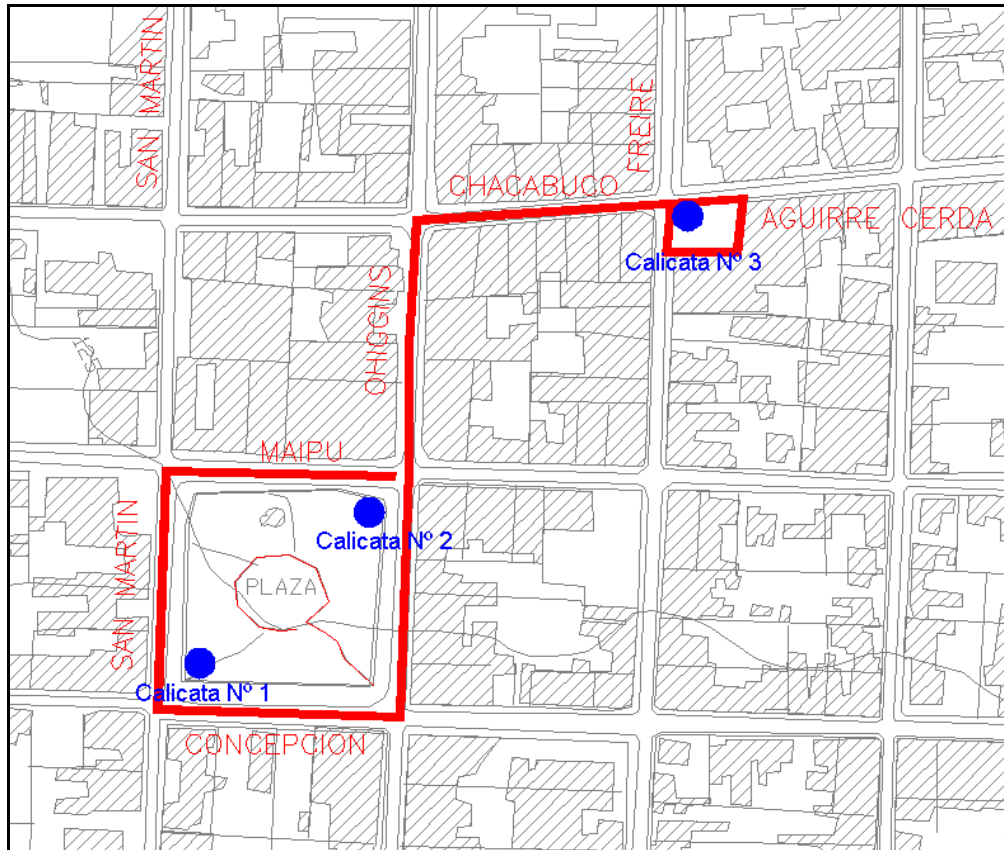
Figura 2. Ubicación calicatas de prospección.
